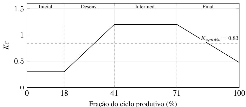
Figura 2. Curva do coeficiente de cultura para o milho, conforme parâmetros cadastrados no sistema (30/40/50/50 dias) e valores FAO-56. A linha tracejada indica o K_c médio ponderado.
