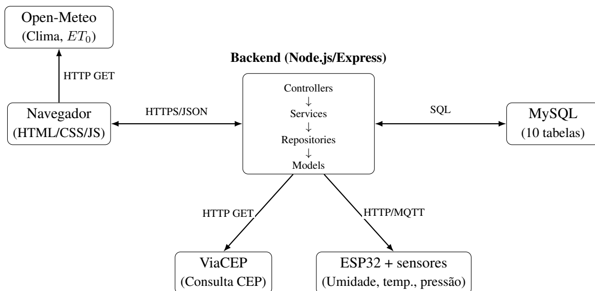
Figura 1. Arquitetura em camadas do TerraFarr. O navegador consome diretamente a API Open-Meteo (HTTP GET) para dados meteorológicos em tempo real, e o backend consome o ViaCEP (HTTP GET) para validação e autopreenchimento de endereços. Dispositivos ESP32 enviam leituras ao backend via HTTP/MQTT.
